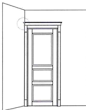
монтаж с недостаточным «приливом»
